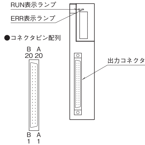
■前面図
